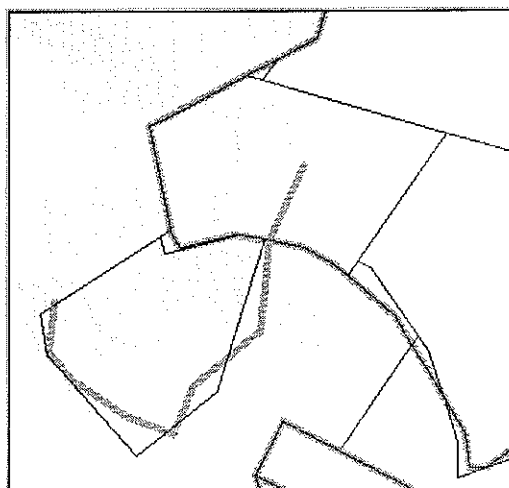
Figura 17: Effetto dell'accorpamento
