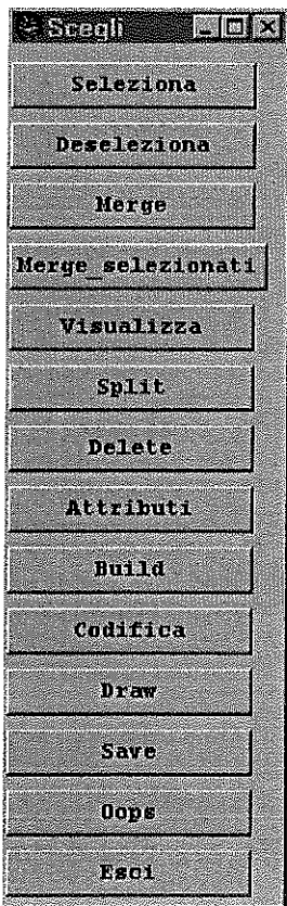
Figura 6: menù "Scegli"
