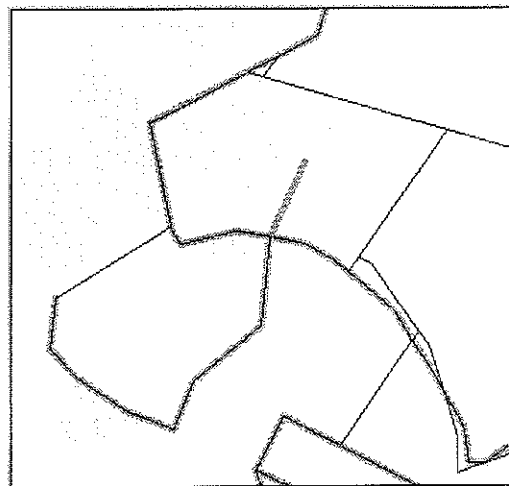
Figura 27: risultato
