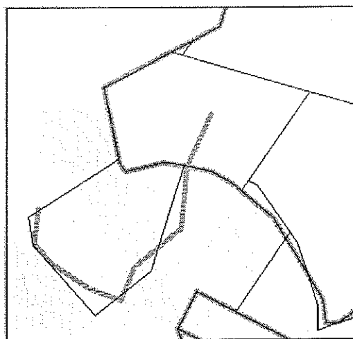
Figura 19: Effetto dell'accorpamento
