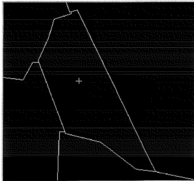
Figura 5: risultato
