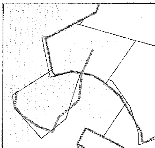
Figura 15: Effetto dell'accorpamento
