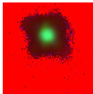
Figura 12. Risposta sonde. Mappa C-scan dei parametri Tv (rosso), A (verde) e S (blu).
