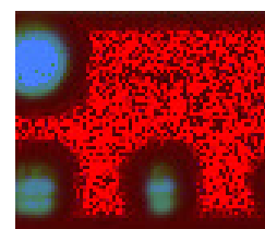
Figura 25. P1. Mappa C-scan dei parametri T_v (rosso), A (verde) e S (blu).
