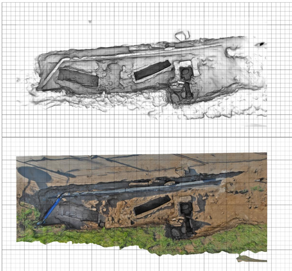
Fig 2 Due rendering del rilievo 3D in visione ortografica con una griglia a 20cm, la semplice geometria del modello acquisito e la versione con texture.
