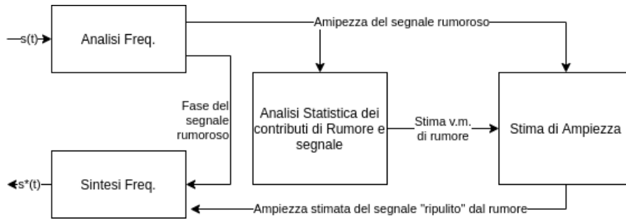
Figura 10: Diagramma a blocchi dell'algorithmo di sottrazione spettrale del rumore
