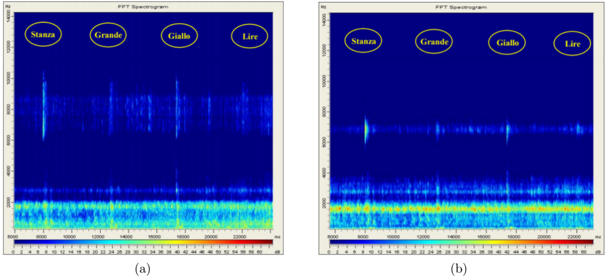
Figura 9: Analisi tempo-spettrale delle parole stanza, grande, giallo, e lire registrata in (a) da un microfono non filtrato e in (b) da una protesi con controllo de rumore [9]
