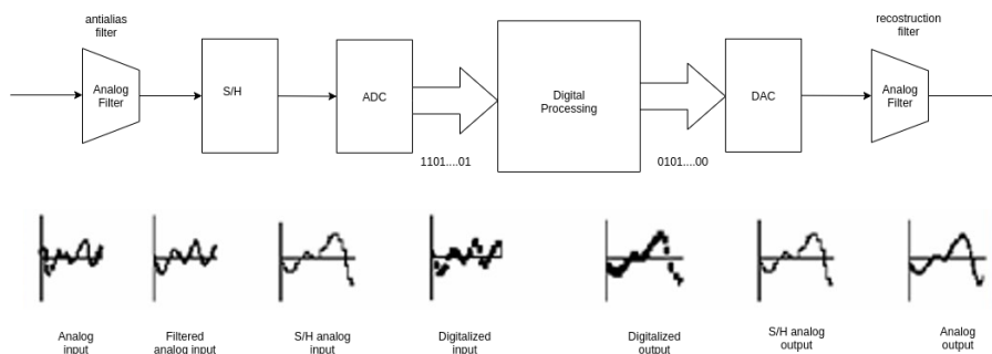
Figura 1: Architettura di un generico sistema di elaborazione digitale di segnali
