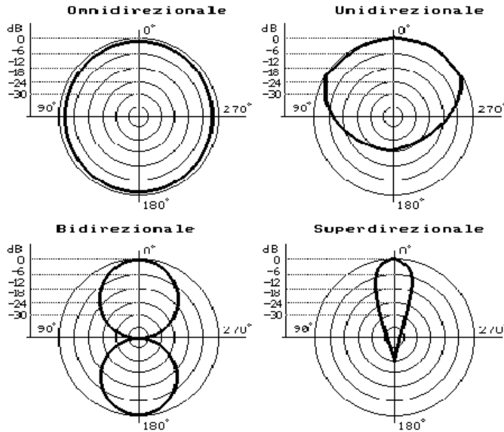
Figura 11: Esempi di diagrammi di direzionalità [9]
