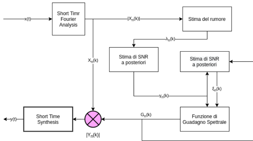
Figura 12: Schema a blocchi che realizza l'algoritmo MMSE
