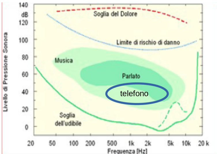
Figura 8: Sovrapposizione di suoni sulle curve isofoniche di Fletcher e Munson
