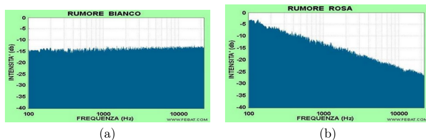
Figura 4: In (a) lo spettro di un rumore bianco, in (b) lo spettro di un rumore rosa
