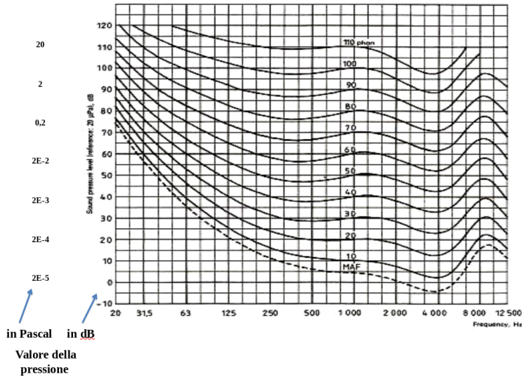
Figura 6: Curve isofoniche di Fletcher e Munson
