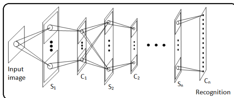
Figura 9: Struttura del Neocognitron. Strati di cellule semplici S e complesse C si alternano
