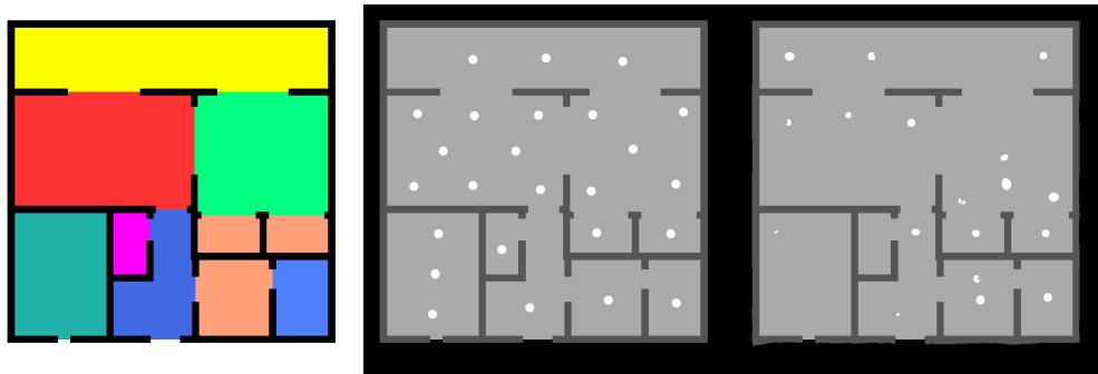
Figura 33: I risultati migliori a questo punto del tirocinio. A sinistra l'input, al centro la mappa target, a destra l'output della rete
