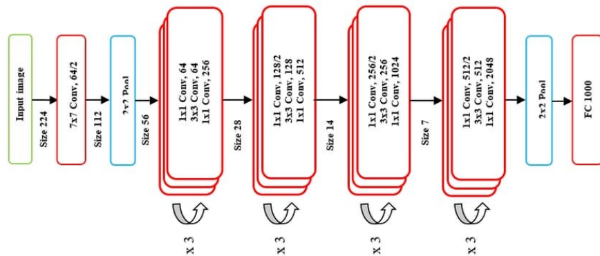
Figura 31: Architettura della ResNet50
