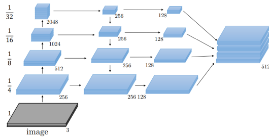
Figura 15: Struttura della Feature Pyramid Network
