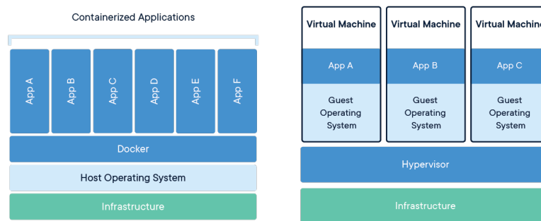
Figura 22: Differenze tra Virtual Machine e Docker
