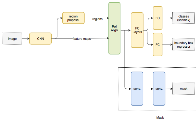
Figura 24: Schema della rete Mask
