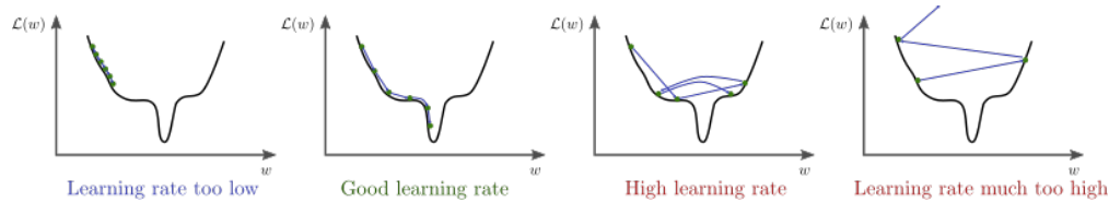
Figura 6: Effetto di diversi learning rate in prossimità di punti di minimo stretti.
