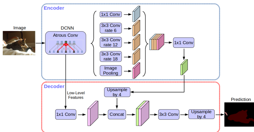
Figura 17: Struttura di DeepLab
