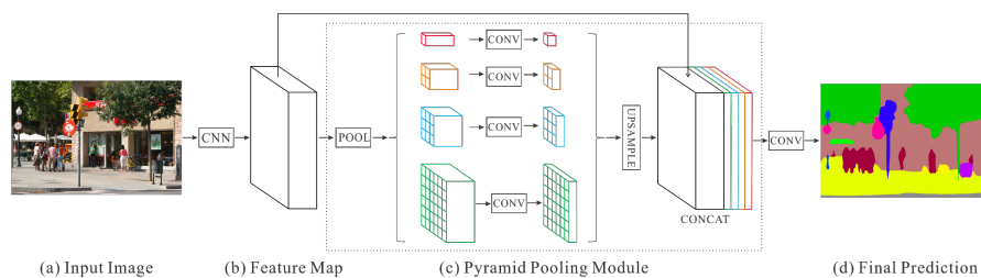
Figura 16: Struttura modello PSP
