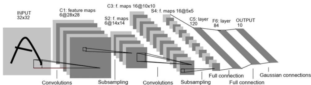
Figura 10: Architettura di LeNet.
