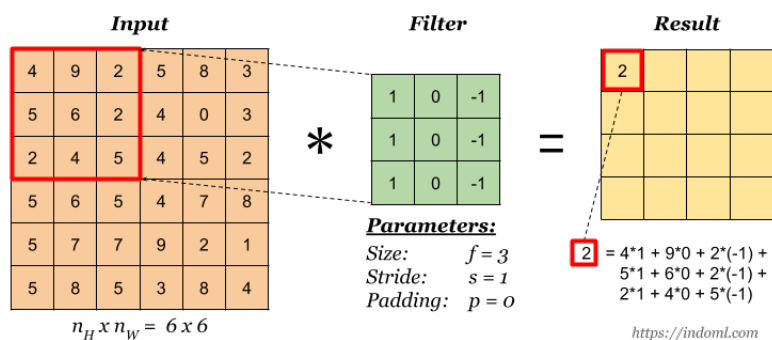
Figura 3: Esempio di convoluzione
