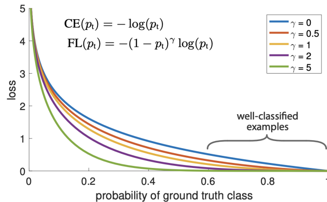
Figura 29: Comportamento della Focal Loss con vari valori di \gamma e pesi standard
