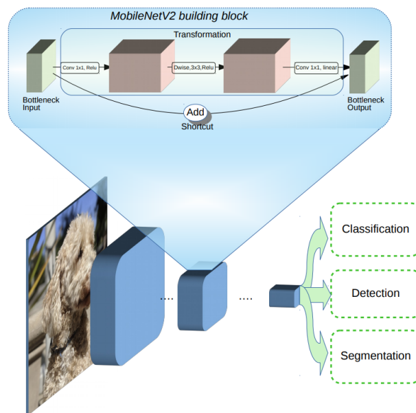
Figura 34: Blocco Convoluzionale della Mobilenet
