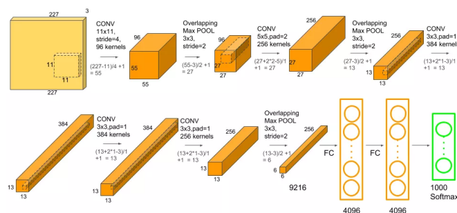
Figura 11: Architettura di AlexNet.
