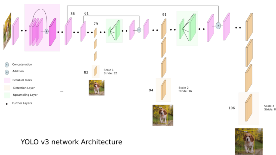
Figura 23: Architettura di Rete di Yolov3
