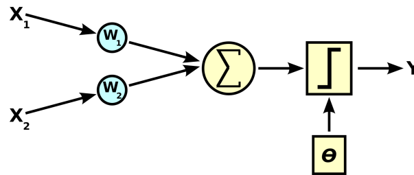
Figura 1: Struttura del Perceptron di Rosenblatt
