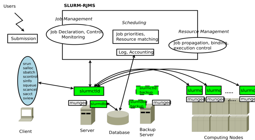
Figura 20: Schema di controllo di Slurm, dalla documentazione ufficiale
