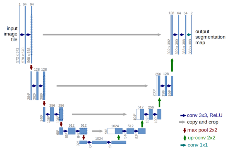
Figura 14: Struttura della UNet Classica
