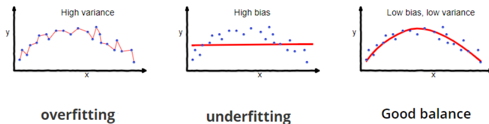
Figura 7: Esempi di overfitting e underfitting in problemi di regressione.
