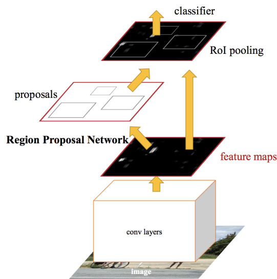
Figura 25: La rete Faster RCNN si basa sull'utilizzo di un Region Proposal Network dopo l'estrazione delle feature
