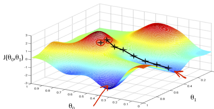
Figura 5: Discesa di gradiente in uno spazio 3D, in evidenza i minimi locali
